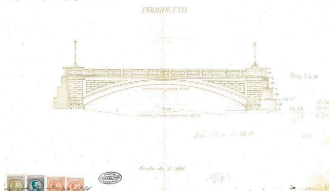
Prospetto del ponte - progetto del 1923
